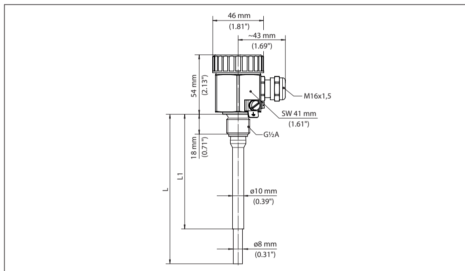
Fig. 7: Sonde de mesure résistive à tige EL 1
